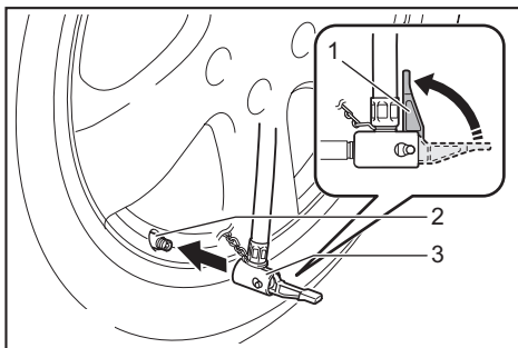
► 1. Pinza del mandril neumático 2. Vástago de válvula 3. Mandril neumático
