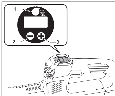
► 1. Unit button 2. Minus button 3. Plus button
